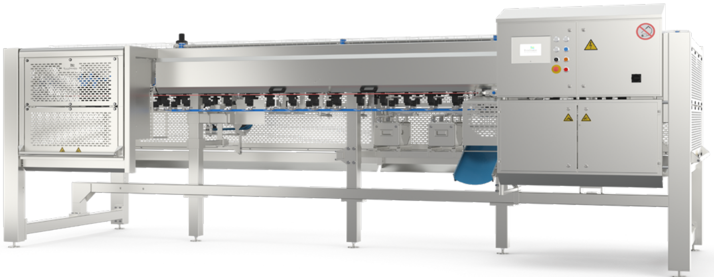
Linienintegrierte Enthäutungseinheit für Oberkeulen
