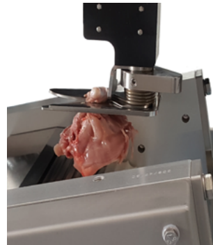
Linienintegrierte Enthäutungseinheit für Oberkeulen
